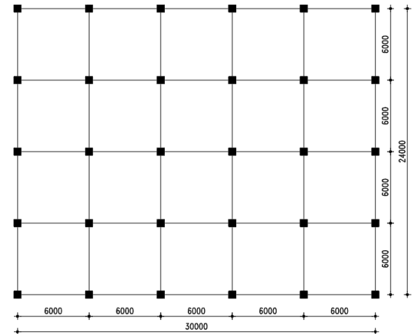
Gambar 3. Denah Gedung Beraturan
